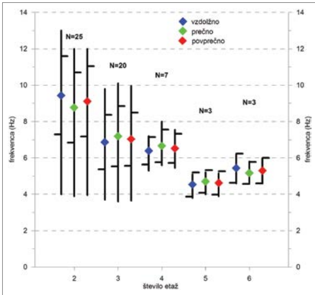
Slika 3: Rezultati statistične analize glavnih frekvenc za 58 analiziranih stavb v odvisnosti od števila etaž (višina). Legenda: rombasti simboli – povprečna vrednost za vzdolžno in prečno smer in njuno povprečje; navpična črta – razpon vrednosti; dve kratki vodoravni črti – povprečje \pm standardni odklon.
