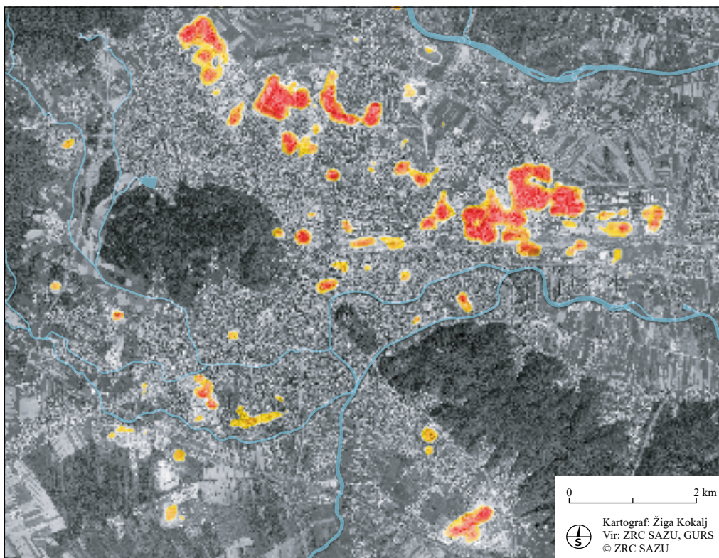
Slika 7: Frekvenca pojavljanja zgornjih dveh odstotkov najvišjih temperatur na pozidanih območjih v Ljubljani. Pozidana zemljišča z veliko toplotno kapaciteto skozi celo leto presegajo povprečne temperaturne vrednosti in se v toplejšem delu leta pogosto pregrevaajo. To so tako imenovane vroče točke. Zemljevid je narejen na osnovi izračuna svetilne temperature tal iz šestih posnetkov termičnega senzorja TIRS na satelitu Landsat 8, ki so bili zajeti med aprilom 2013 in marcem 2014 (Cedilnik, Oštir in Kokalj 2016).
