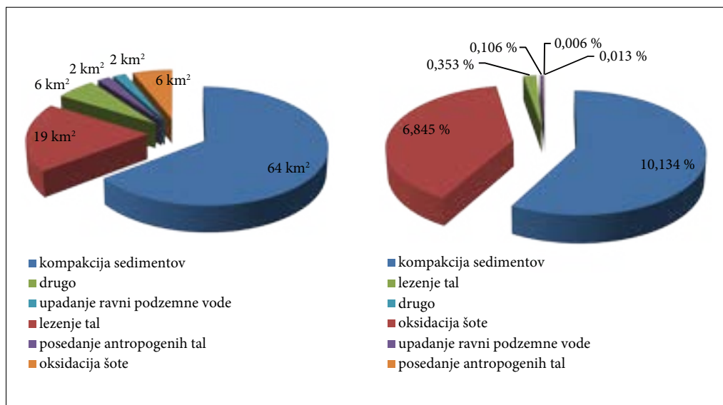
Slika 2: Porazdelitev različnih vzrokov posevanja tal; levo po velikosti območij v km², desno po deležu vzrokov posevanja.
