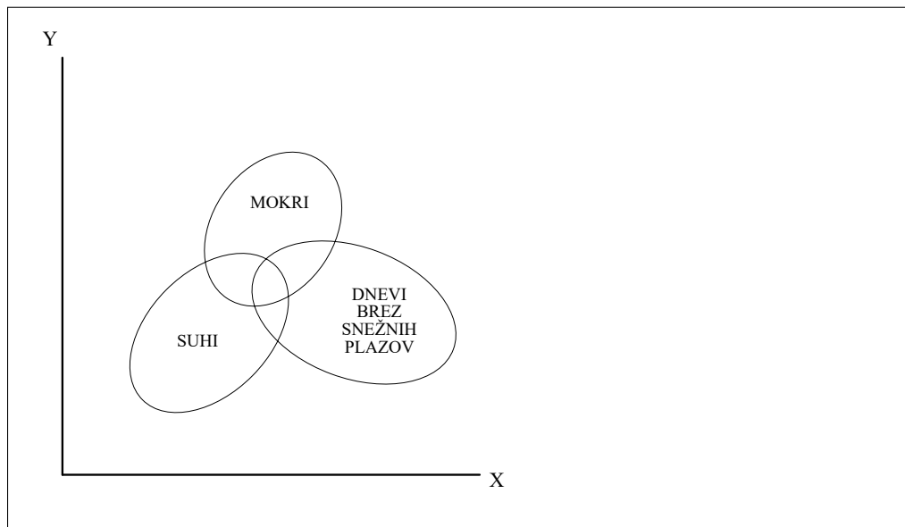
Slika 1: Prikaz dni, ko so se pojavljali snežni plazovi (mokri, suhi) in dnevi, ko snežnih plazov ni bilo, kot primer razvrščanja primerov po diskriminantni analizi (McClung in Schaerer 2006).
