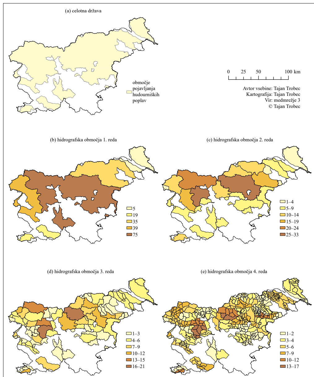
Slika 2: Razporeditev in število hudourniških poplav po hidrografskih območjih različnih redov v Sloveniji za obdobje 1951–2015.
