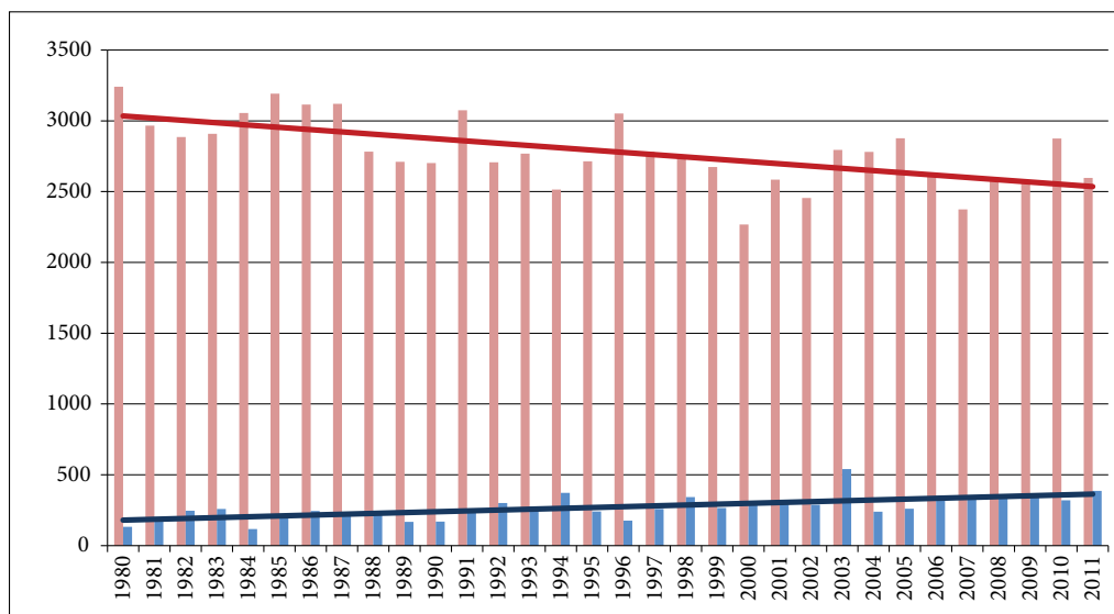
Slika 6: Vsota stopinjskih dni ( ^{\circ}\text{C} ) za ogrevanje (rdeča) in ohlajanje (modra) v Ljubljani (Komac s sodelavci 2016).
