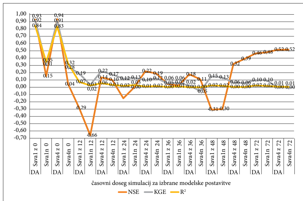
Slika 4: Merila (NSE, KGE, R^2 ) kakovosti napovedi pri pretokih nad 100 \text{ m}^3/\text{s} s povečevanjem časovnega dosega za izbrane modelske zasnove za obdobje 14. 1. 2014–29. 02. 2016, vodomerna postaja Sora Suha.
