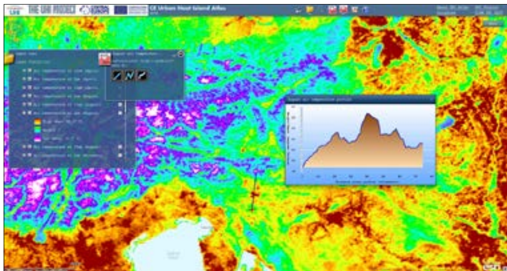
Slika 8: Atlas mestnega toplotnega otoka za Srednjo Evropo.
