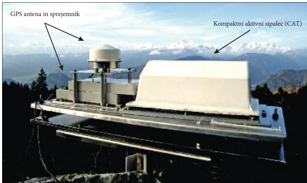
Slika 1: I2GPS enoto sestavlja GPS sprejemnik in antena ter CAT.
