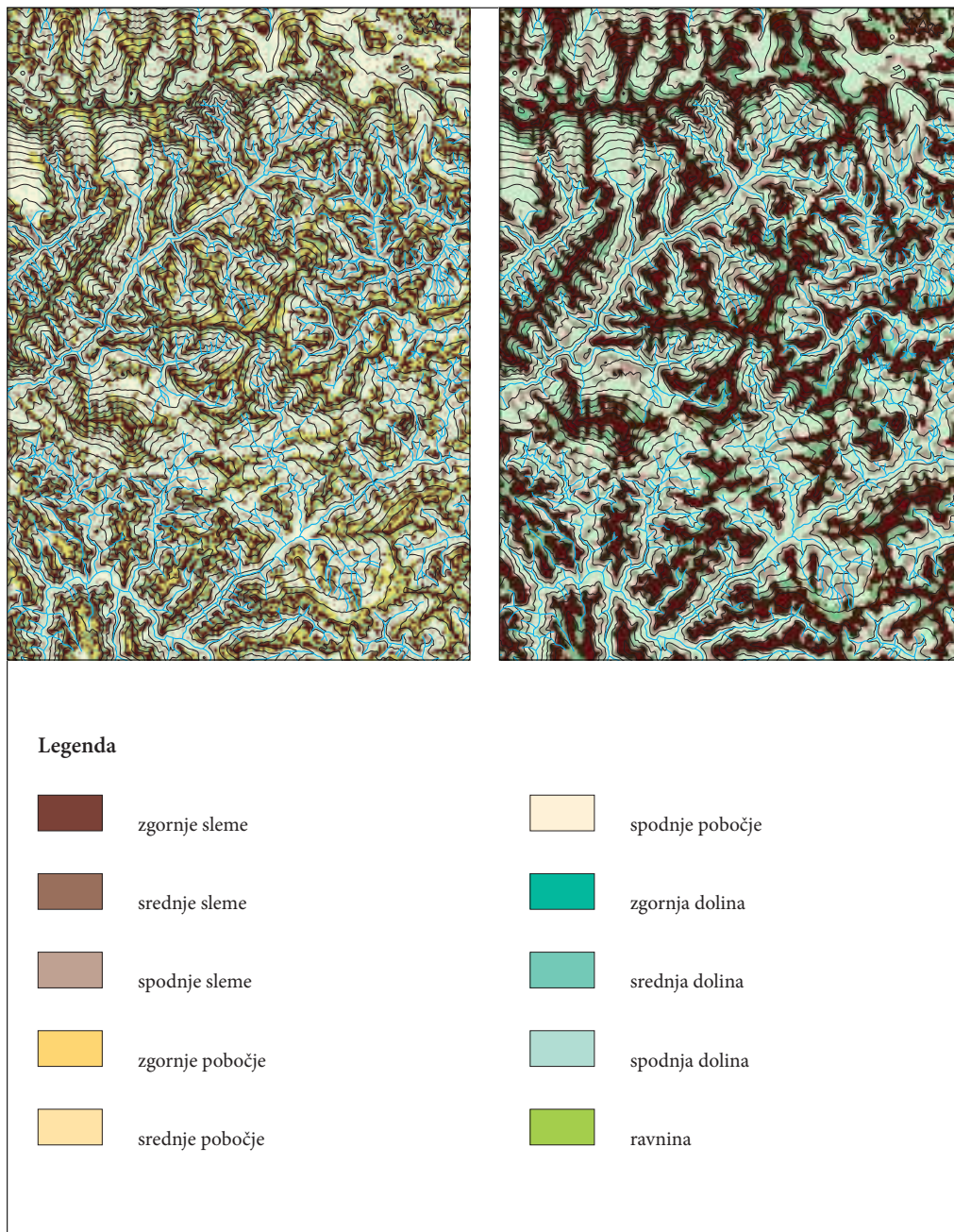
Slika 1: Razlike med morfološkimi enotami površja okoli Porezna zaradi različnih kombinacij obsega sosedstva. Levo so morfološke enote določene s kombinacijo stometrskega in devetstometrskega sosedstva, desno pa s kombinacijo petstometrskega in dvatisočmetrskega sosedstva.
