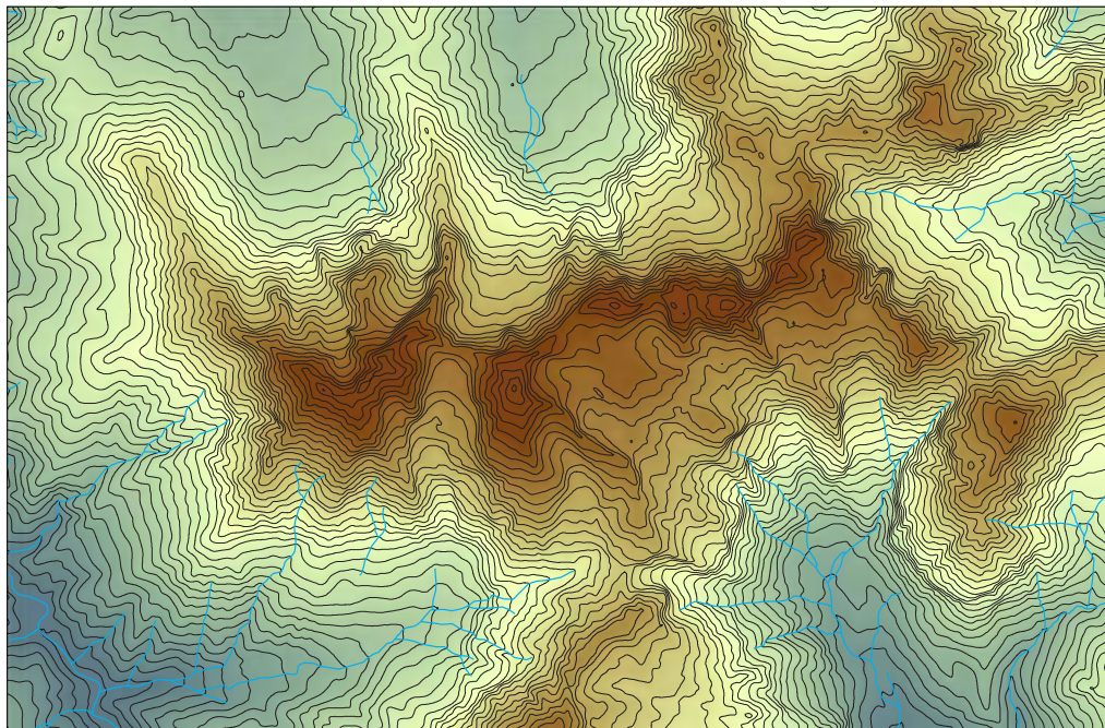
Slika 3: Višine površja v območju Kamniško-Savinjskih Alp.
